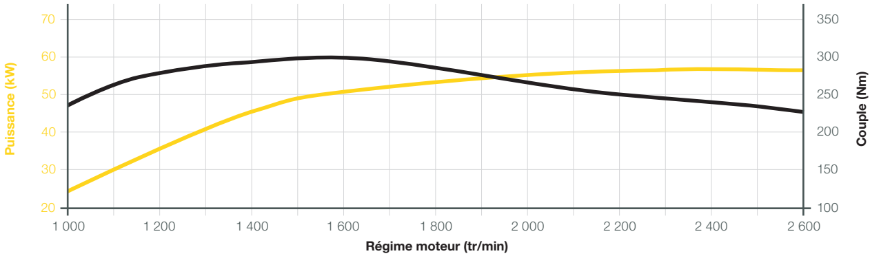
Caractéristiques de puissance du moteur KDI 2504 TCR ; 55,4 kW ; phase V
