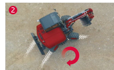
2 Direction sur les quatre roues Petit rayon de braquage sur les chantiers étroits
